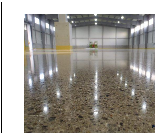
3-расм. Мрамар увоқларидан бетонли полларни қуриш
