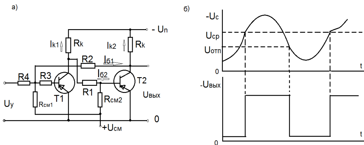
Рис.1. Схема (а) и диаграмма работы (б) реле на транзисторах.
