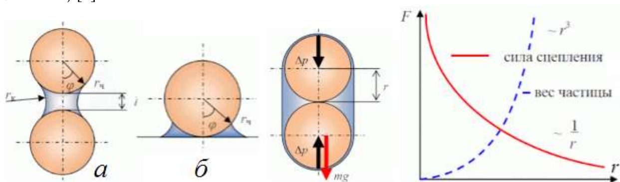
Рисунок 1 – Образование капиллярного мениска: между двумя сферическими частицами (а); между сферической частицей и плоскостью, (б) Схема капиллярного сцепления двух шарообразных песчинок, с) Зависимость силы поверхностного натяжения от радиуса частиц.
