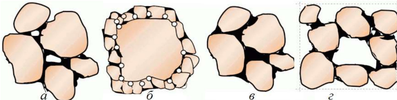
Рисунок 4 – Капиллярные структуры в дисперсных системах: а – трехфазная гранула; б – трехфазная глобула; в – двухфазная гранула; г – ячеисто-глобулярная структура.
