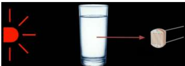
Рис. 2. Мутность обусловлена рассеянием световых волн.
