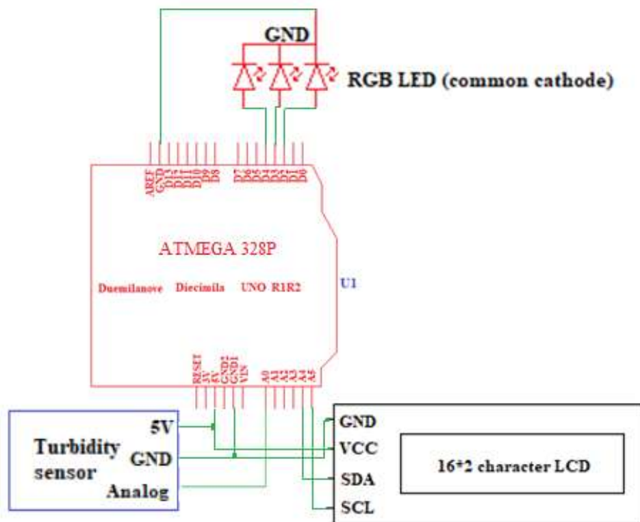
Рис. 5. Схема подключения Arduino с датчиком мутности.
