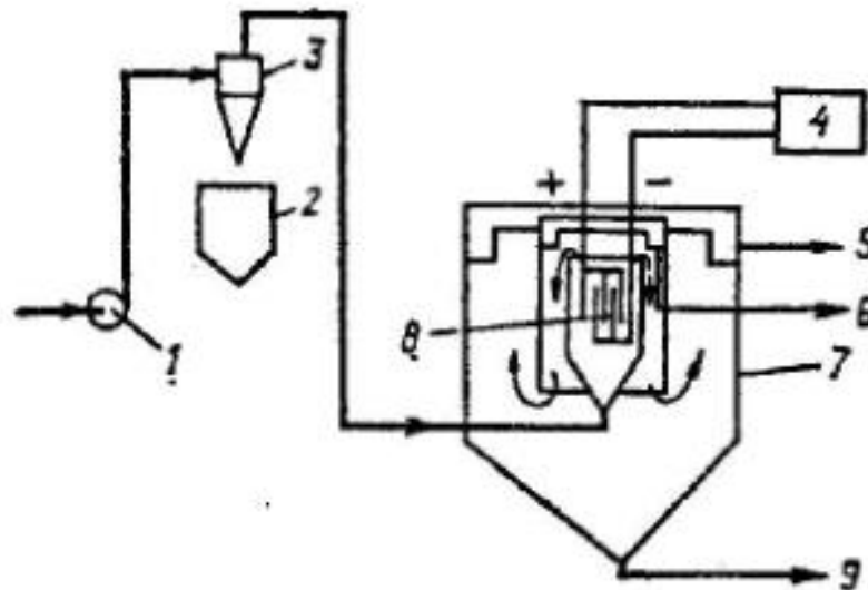
Рис.1. Установка электрокоагуляционной очистки.
