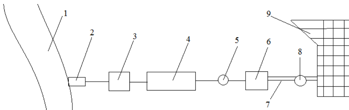
Рис.2. Схема водоснабжения.
