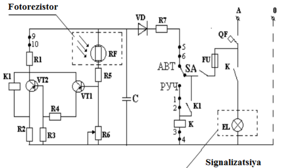
Rasm.1. Loyqalangan suvni chegarasini avtomatik nazorat qilish qurilmasini prinsipial sxemasi.
