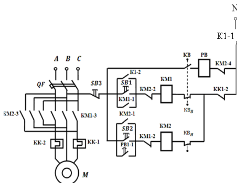
Rasm. 2. Zatlarni ishga tushirish sxemasi.
