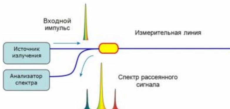
Рис.1. Схема на основе эффекта КР.
