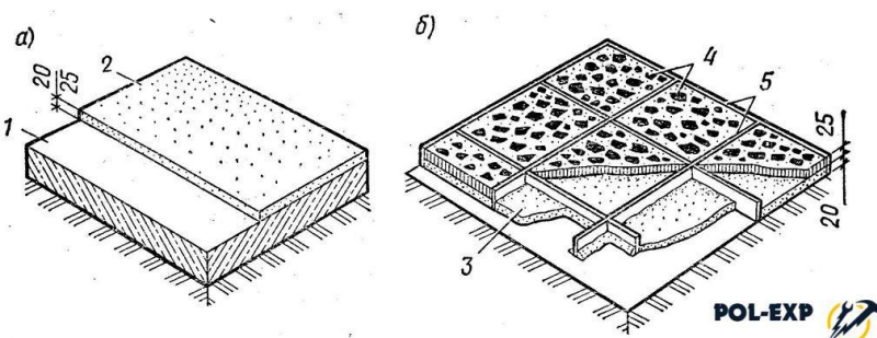
5-расм. Грунт устига жойлаштирилган цементли ва мрамар поллар
