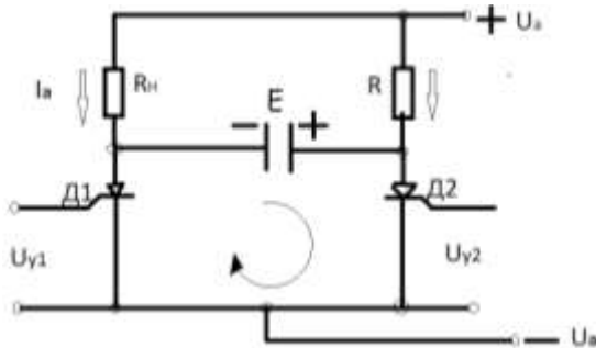
Рис. 2. Схема тиристорного реле.
