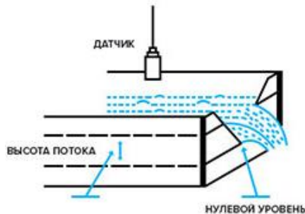
Рис.4. Треугольный водослив.
